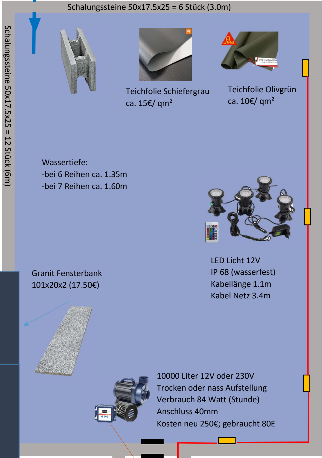
Pumpe und LED Licht 12V Elektrik im Schacht
